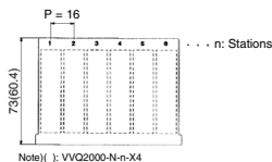
Note) (-): VVQ2000-N-n-X4
