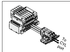
Double check block VQ1000-FPG-□□-□
