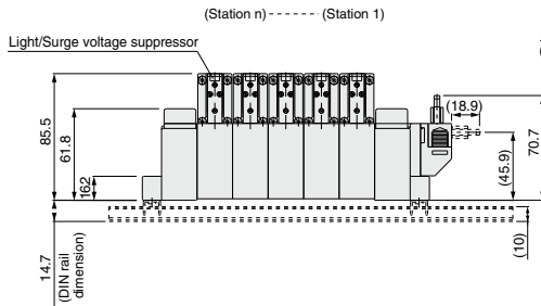
10PG (20 pins)
